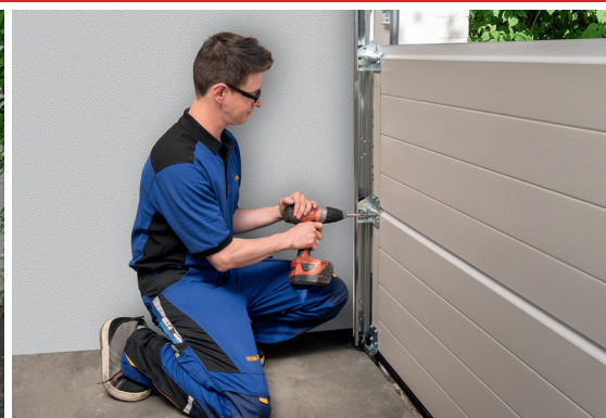
Fachgerechte Montage
